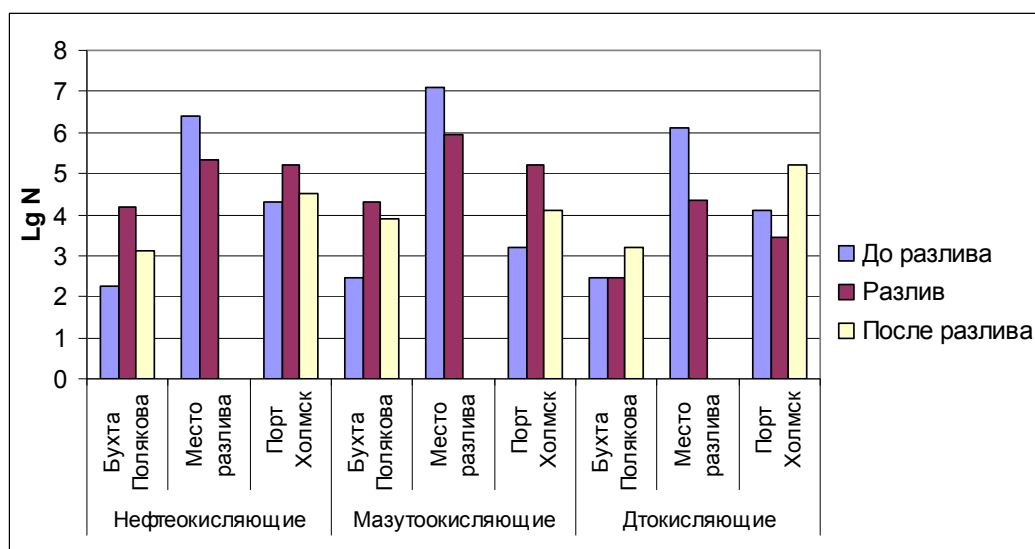
Рис. 3. Численность НУО микроорганизмов в морской воде при крушении судна «Христофор Колумб» в районе г. Холмска в сентябре 2004 г. (N – кл/мл)
