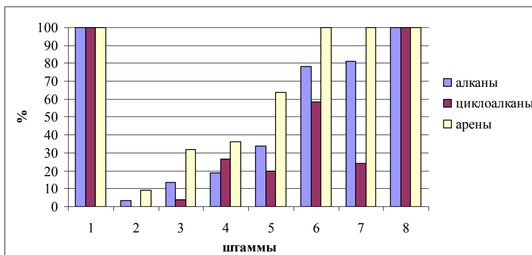
Рис. 4. Утилизация НУ бактериями разных физиологических групп за 30 суток. 1 – контроль, 2 – штамм 59 (++++), 3 – штамм 8 (++++), 4 – штамм 21 (+++), 5 – штамм 410 (+++), 6 – штамм 10 (++) , 7 – штамм 81 (+++), 8 – штамм 73(+)
