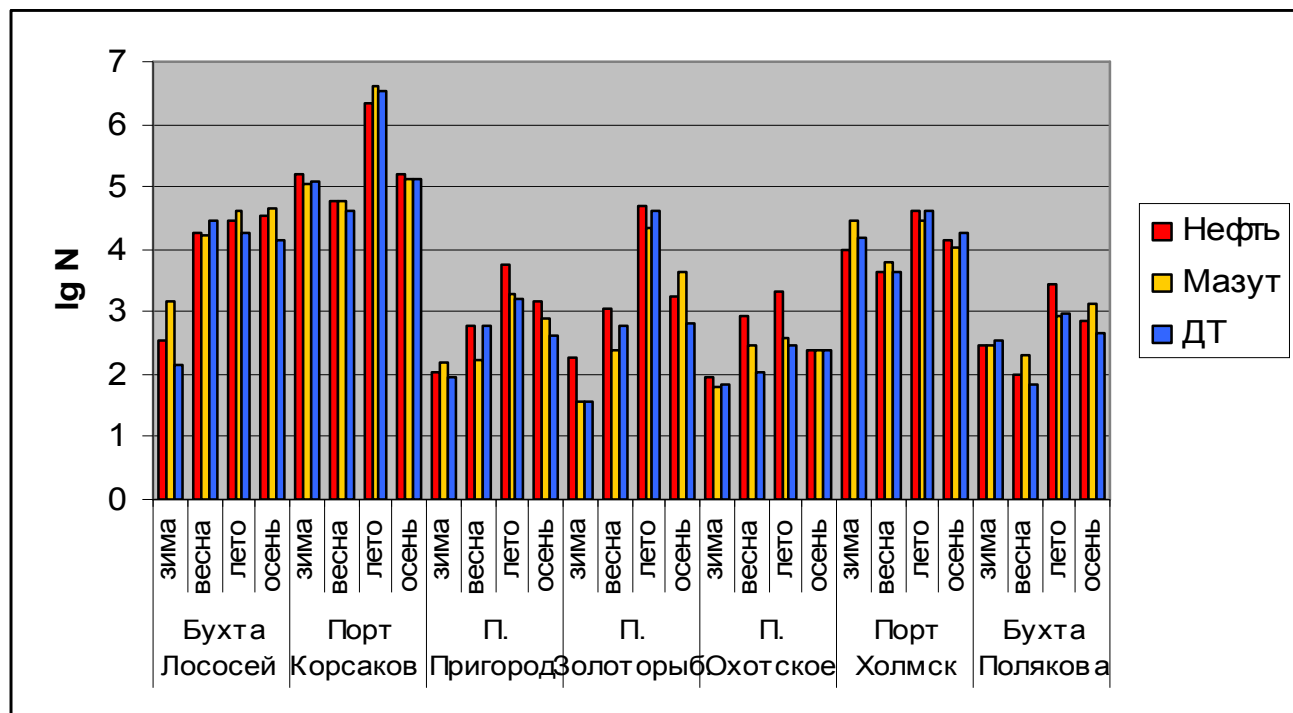
Рис. 2. Изменение средней численности НУО микрофлоры в морской воде по сезонам в 2004-2006 гг. (N – кл/мл)
