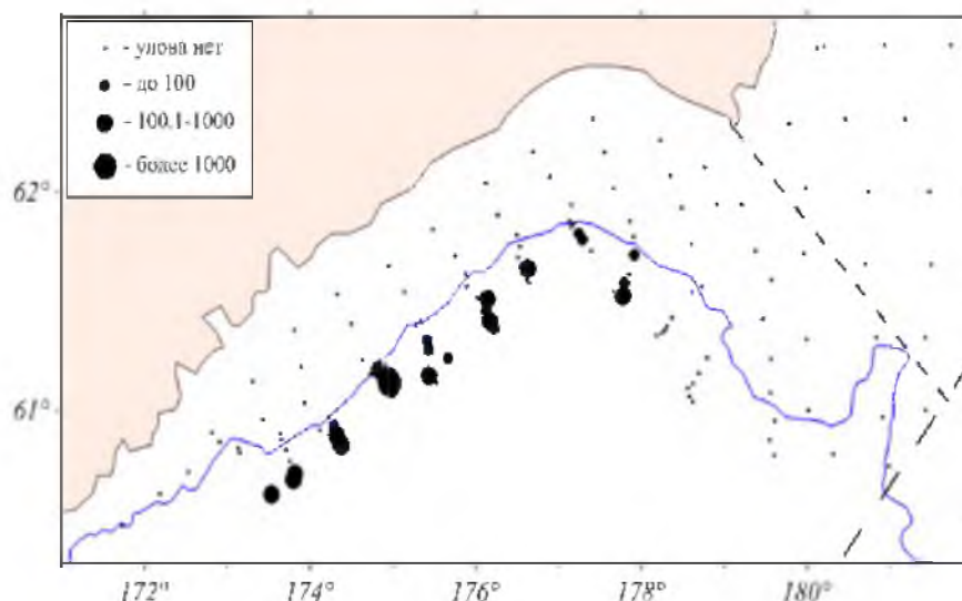
Рис. 11. Распределение плотности S. alascanus в Олюторско-Наваринском районе Западно-Беринговоморской зоны летом 2015 г., экз./км 2
