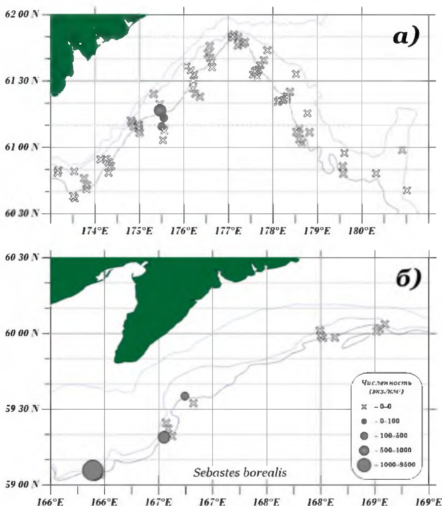
Рис. 4. Распределение численности северного морского окуня на Корякском (а) и Карагинском (б) свалах глубин материкового склона Берингова моря в августе–сентябре 2024 г.
