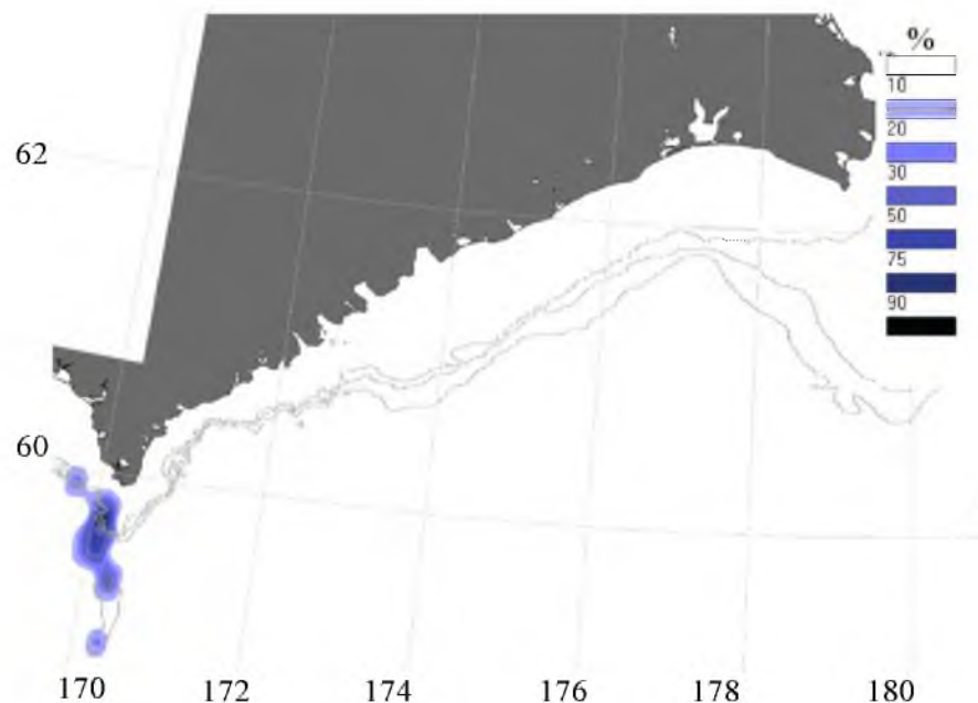
Рис. 2. Осредненное распределение уловов терпуга при специализированном промысле пелагическими травами в Западно-Беринговоморской зоне (в % от максимальной плотности). По данным ИСР «Рыболовство» за 2010-2020 гг.
