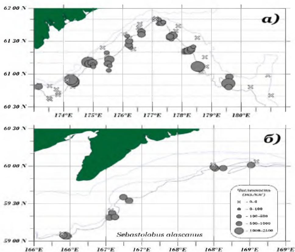
Рис. 14. Распределение численности аляскинского шипощека на Корякском (а) и Карагинском (б) свалах глубин материкового склона Берингова моря в августе–сентябре 2024 г.
