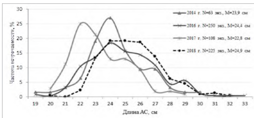
Рис. 47. Размерный состав омуля Штейндахнера в Кунаширском проливе в сетных уловах 2014, 2016–2018 гг. (M - ср. длина, N - кол-во промеренных особей)
