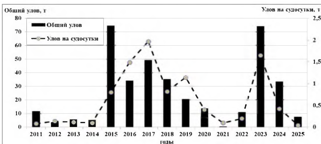
Рис. 3. Динамика количества судосуток и уловов на судосутки при донном ярусном промысле морских окуней в Западно-Беринговоморской зоне в 2011–2025 гг.
